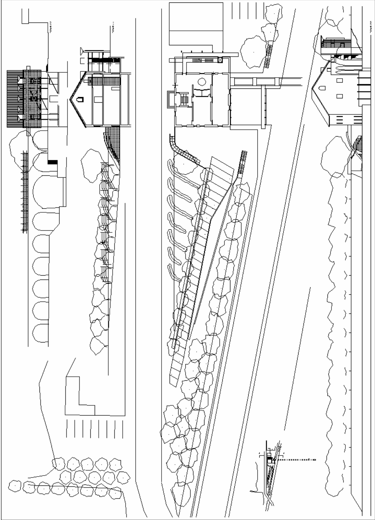
Plan. e Prospetti edificio Sollevatore delle acque
